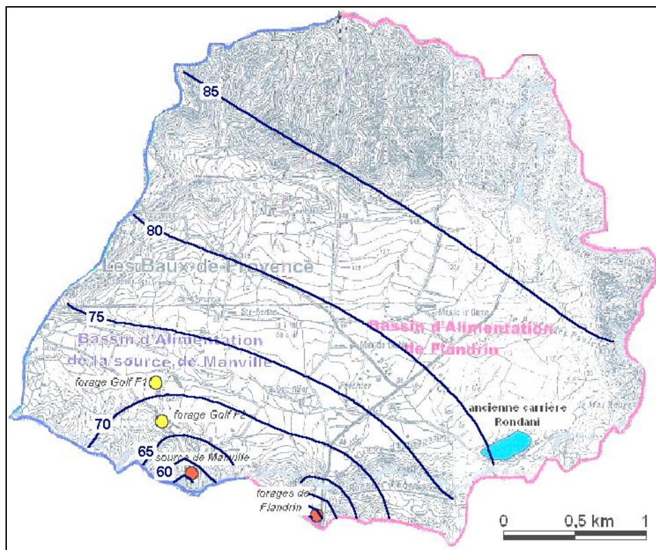
Piézométrie simulée avec les prélèvements existant sur le secteur
